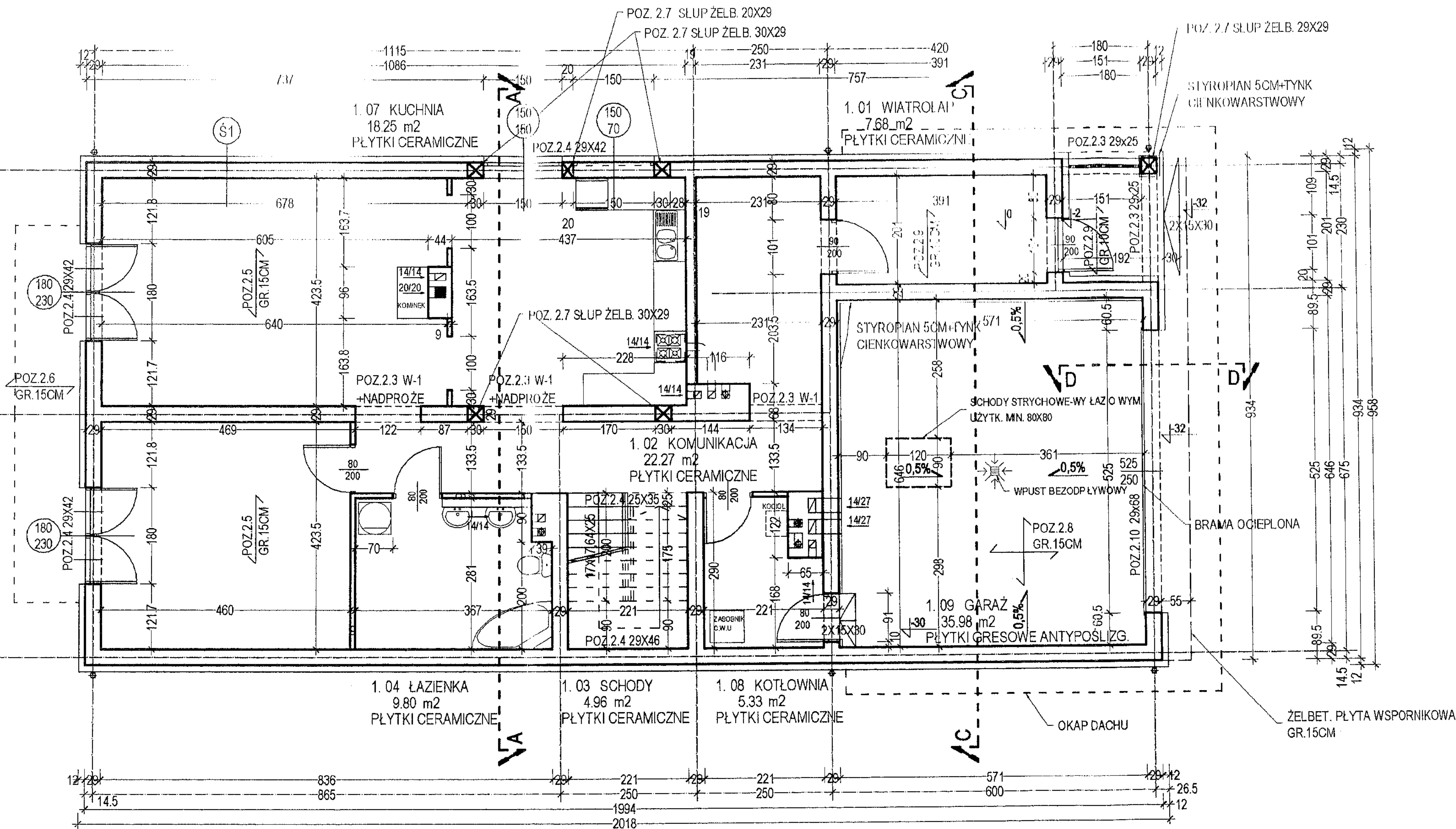
RZUT PARTERU SKALA 1:100
