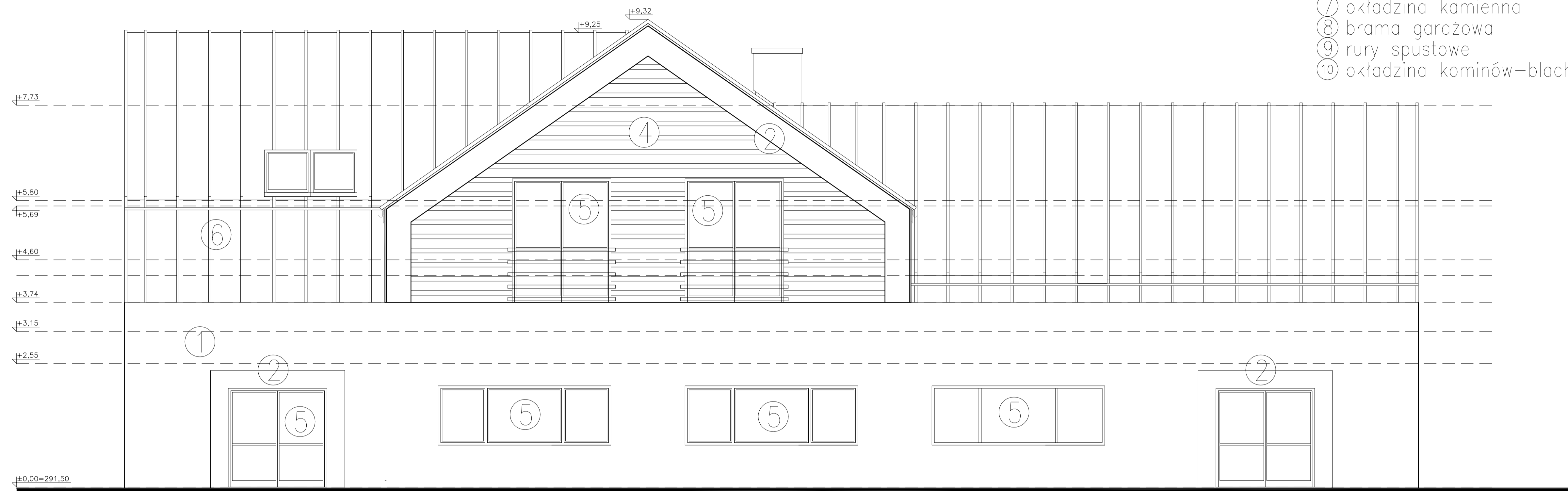
elewacja południowa
